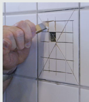
Skär ett spår langs plattkanter. Avlägsna plattan försiktigt
